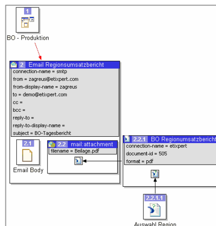
Abb.2: Einfache Integration der BO-Funktionalität
